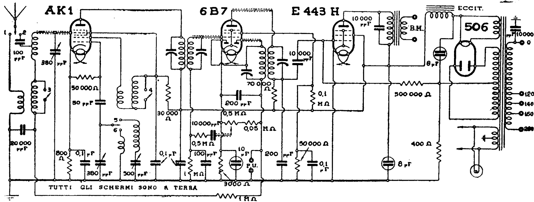
WATT RADIO . MOD. « ERMETE »
